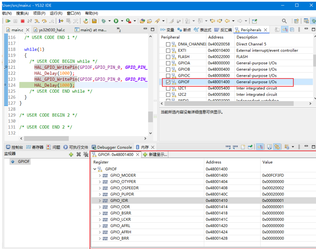
图 4-18 查看外设寄存器
